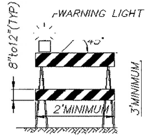
TYPE II BARRICADE
